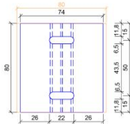
Lochdurchmesser 6,5mm holepattern 6,5mm
